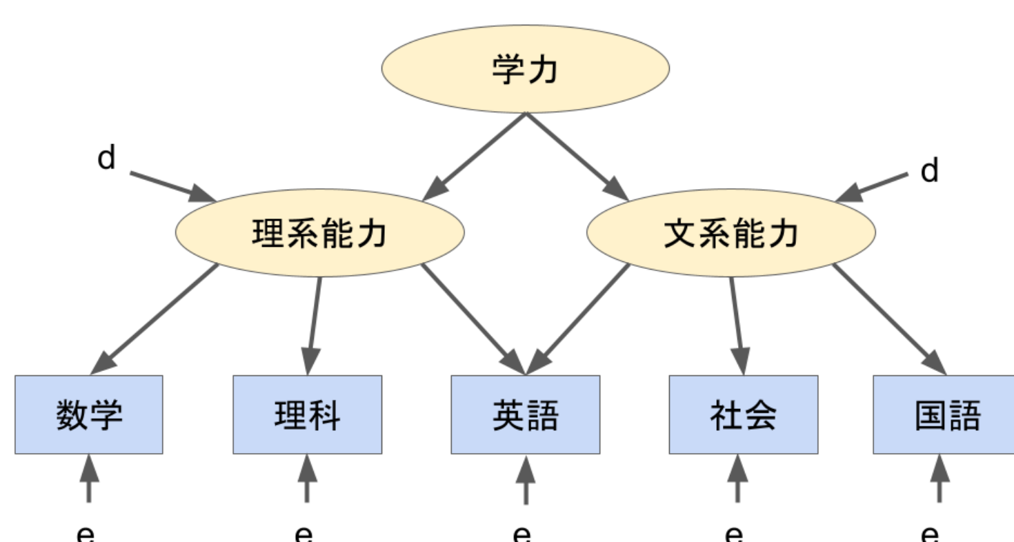
構造方程式モデリングの例
