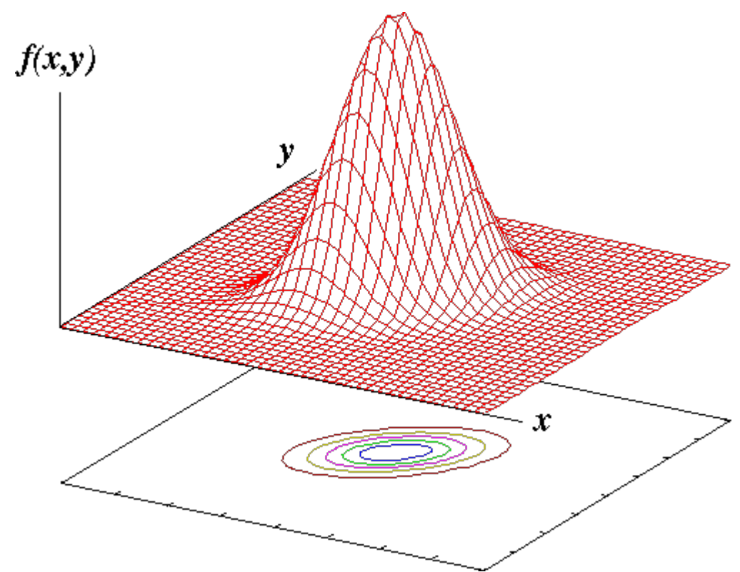
多次元正規分布のグラフ
